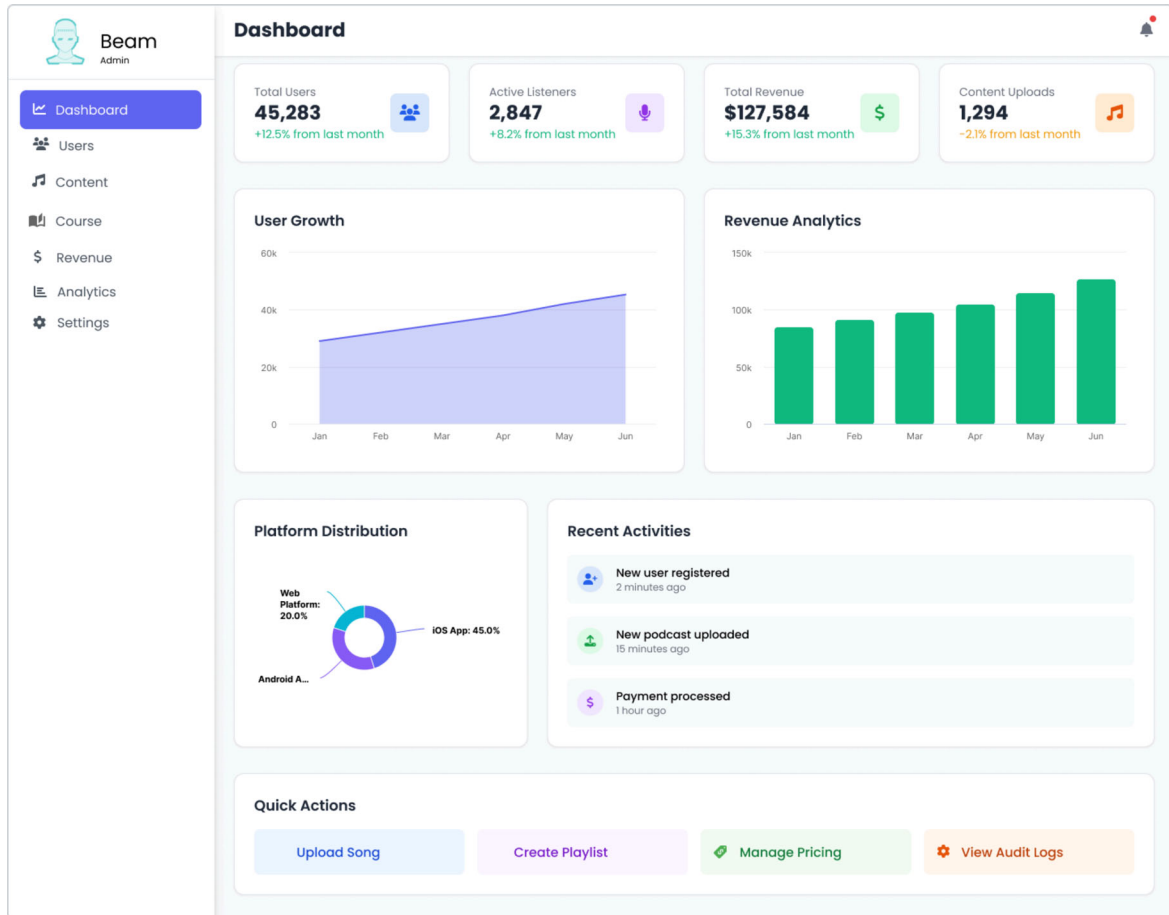
รูปภาพแสดงหน้า Admin Dashboards
